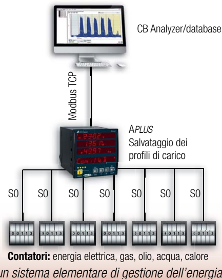
Analisi del profilo di carico con il software CB Analyzer
