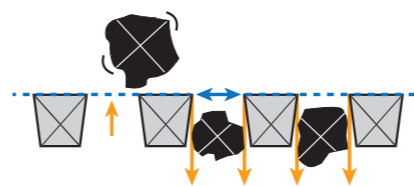
Des ouvertures coniques empêchent le colmatage. Le fond du tamis reste propre.
