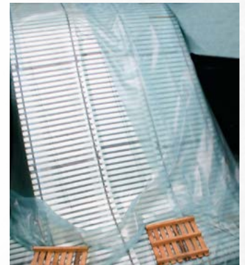
Details: Kunststoffrohre 80x30x2 in 2 Gurtbändern verschraubt Gesamtabmessung: ca. 2.150x1.500x35mm (LxBxH)
