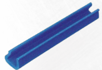
Details: PE-Schaum Farbe: blau Standardlänge: 2m ±2% Lichtes Innenmaß: max. 92mm Materialstärke: 18mm Verpackungseinheit: 72m
