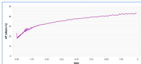
Facteur d'antenne HyperLOG 3080
