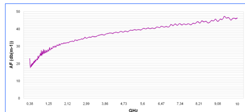
Facteur d'antenne HyperLOG 30100
