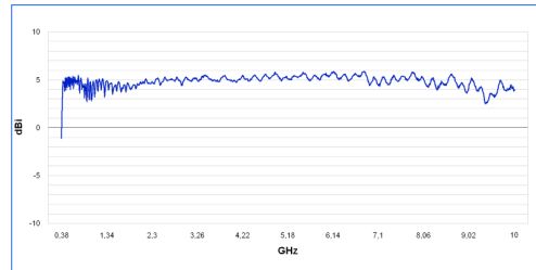
Diagramme de gain HyperLOG 30100
