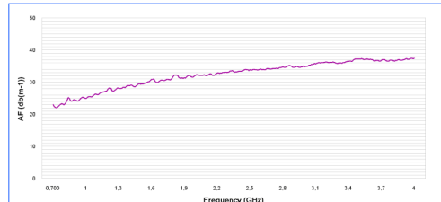
Antennenfaktor HyperLOG 7040
