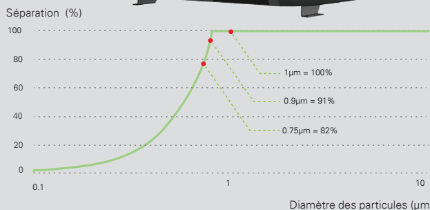
Schéma: Le tableau montre l'efficacité de nos épurateurs selon le diamètre des particules aspirées, au débit nominal.
