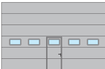
SPU F42 Lamellenfenster Typ E Schlupftüranordnung Mitte
