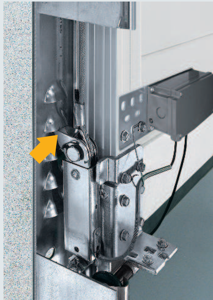
Der Verriegelungshaken der Aufschiebesicherung rastet beim Hochhebeln des Tores automatisch fest ein.
