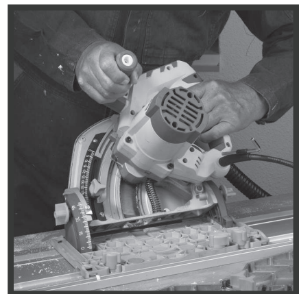
Doppel Vorder- und Hinterachse für genaue und präzise Schnitte.
