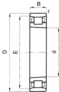
N10KTN
