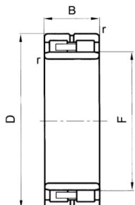
NNU49B/G
