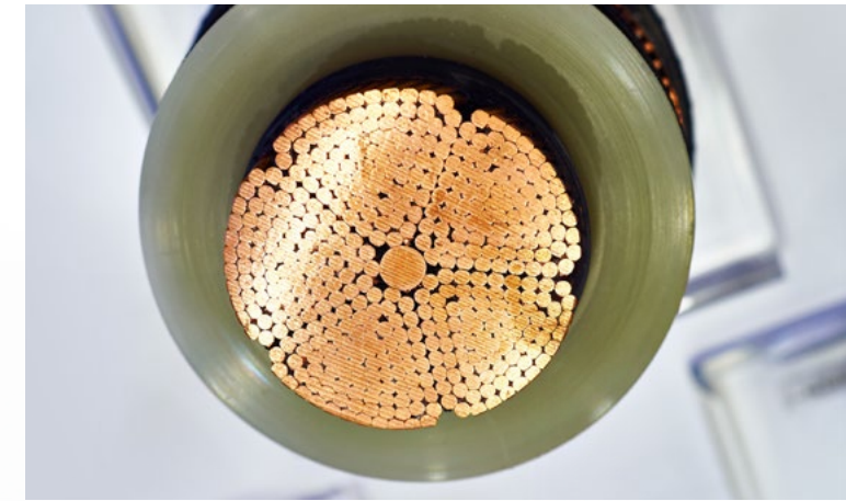
Kontaktieren mit FrontCon: Kein Abisolieren der Einzeldrähte.
