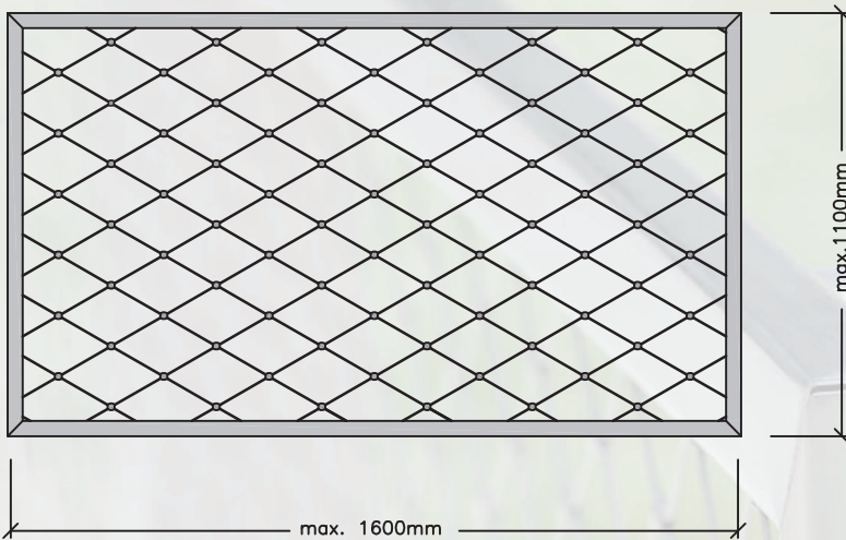
Carl Stahl X-TEND3 liegende Maschenrichtung horizontal mesh diamond direction
