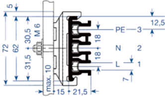
Montaje lateral
