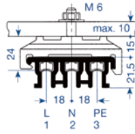
Montaje suspendido
