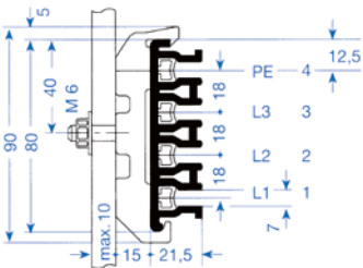
Montaje lateral
