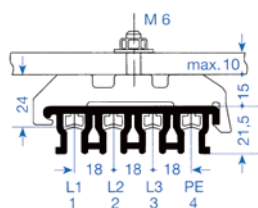
Montaje suspendido
