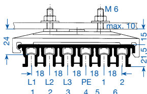
Montaje suspendido
