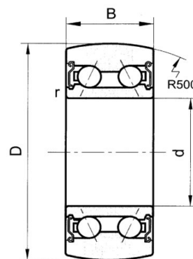
LR52A-ZZ LR53A-ZZ
