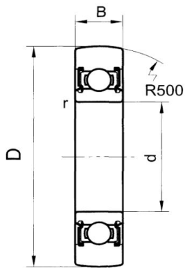
LR1A-2RS LR2A-2RS
