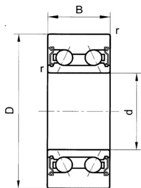
LR52-ZZ LR53-ZZ
