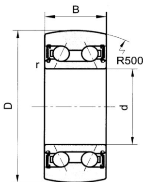
LR52A-2RS LR53A-2RS
