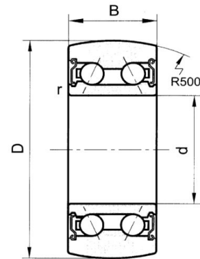
LR52A-ZZ LR53A-ZZ
