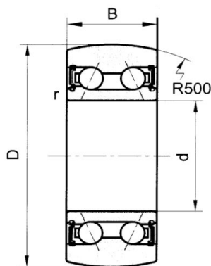
LR52A-2RS LR53A-2RS
