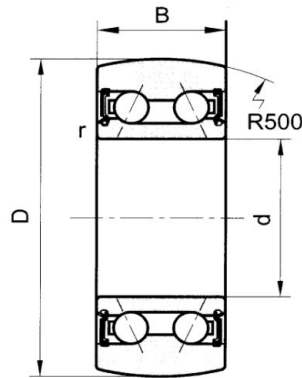
LR52A-2RS LR53A-2RS
