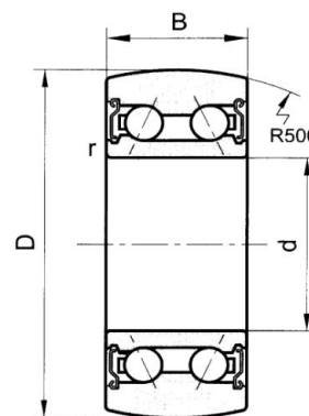
LR52A-ZZ LR53A-ZZ
