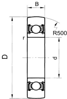
LR1A-2RS LR2A-2RS
