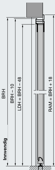
Sidedør med alu-hjørnekarm profiltype 2 Utvendig montering
