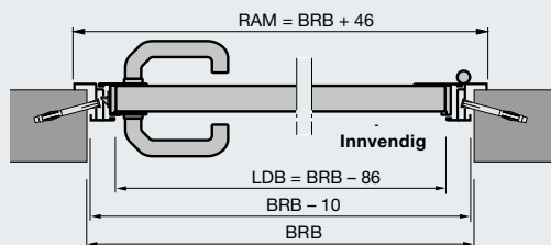
Sidedør med alu-hjørnekarm profiltype 3 Utvendig montering
