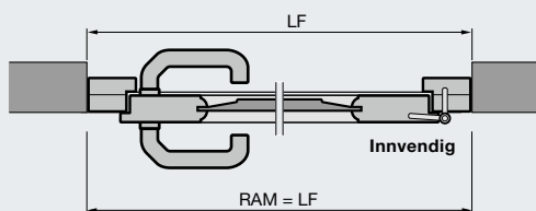
Sidedør i massivt tre Montering i åpningen
