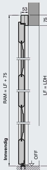
Sidedør i massivt tre Montering bak åpningen
