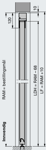
Sidedør med alu-blokkarm, profiltype 2 Montering i åpningen
