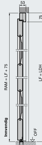
Sidedør i massivt tre Montering i åpningen
