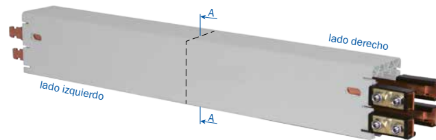
KBHS con junta de unión por tornillos
