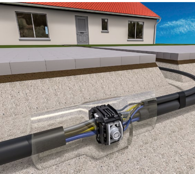
ISICOMPACT: Zuverlässiger Hausanschluss mit nur einer Schraube.
