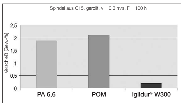
Abb. 67.2: Verschleiß bei 100 N Axiallast auf TR20x4-Gewinde. Spindel und Trapezgewindemuttern wurden vor dem Versuch gereinigt und entfettet
