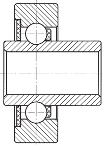
Laufrolle einseitig gedichtet, mit verlängertem Innenring.
