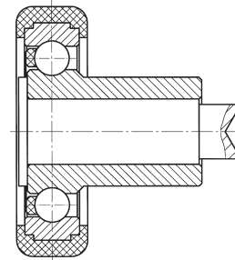
Laufrolle mit integriertem Bolzen und Delrin-Ummantelung
