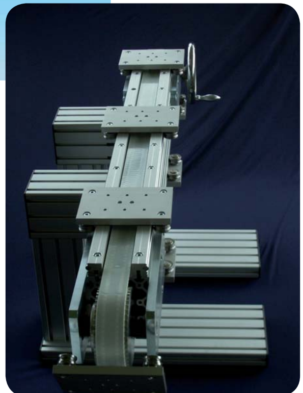
(Messemodell mit Handrad)
