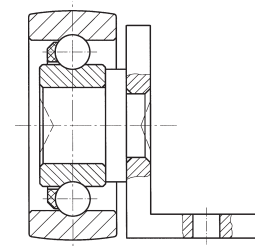
Laufrollen-Unit mit profiliertem Aussenring, mit Halterung über verstemmten Bolzen an einem verzinkten Winkelblech
