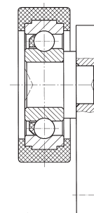
Laufrollen-Einheit mit kunststoffummantelter Laufrolle, Befestigung über vernieteten Bolzen in einer Stahlplatte.
