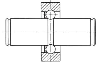
Laufrolle mit integriertem Bolzen und Sicherungsnuten
