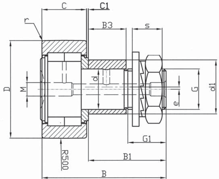
fehlende Maße siehe Seite 48/49.
