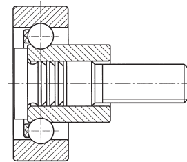
Laufrolle mit integriertem Gewindezapfen
