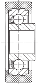
Laufrolle mit Desmopan-Ummantelung, mit verlängertem Innenring.
