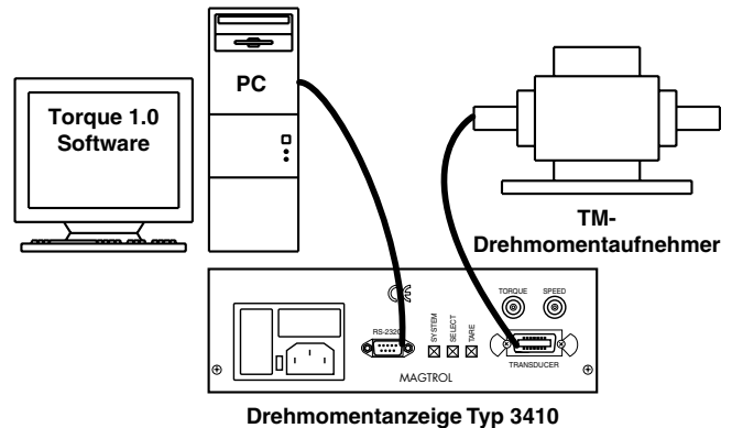
Systemkonfiguration mit PC Drehmomentmesswelle mit Anzeigegerät Typ 3410 und Torque 1.0 Software
