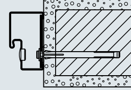
Tam kasa Örme duvara montaj Dübel montajı
