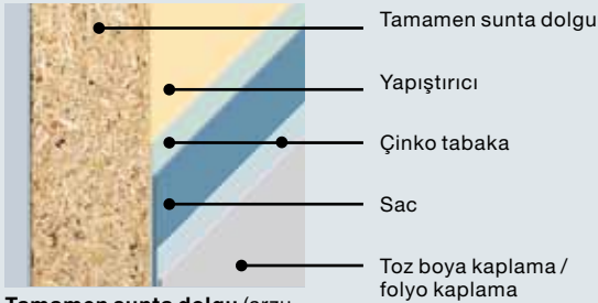
Tamamen sunta dolgu (arzu edilirse) daha iyi ses koruması için
