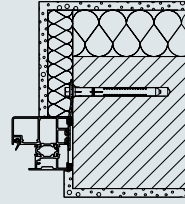
Tam kasa Ankrajlı montaj
