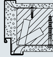
Tam kasa Örme duvara montaj Duvar dübel ankrajı
