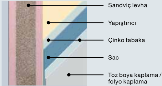
Sandviç levha
