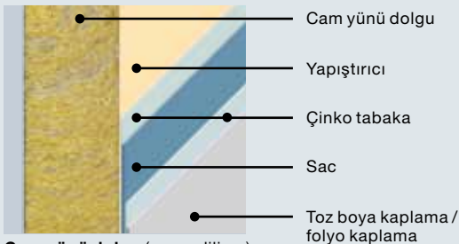
Cam yünü dolgu (arzu edilirse) daha iyi ısı yalıtımı için
