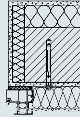
Tam kasa Açıklığın arkasına montaj (sadece MZ Thermo)
