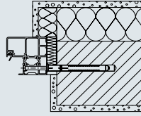
Tam kasa Örme duvara montaj Çerçeve montajı
