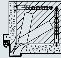
Köşeli kasa Örme duvara montaj Duvar dübel ankrajı
