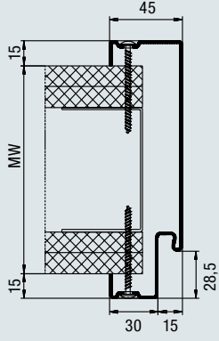
Profil 21120 Vidalanan ayna bağlantısı
