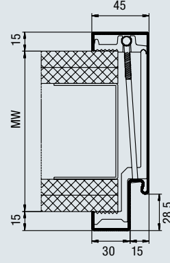
Profil 21120 Sıkıştırılmalı sabitleme
