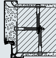
Köşe ve ilave kasa Dübel ankraj montajı
